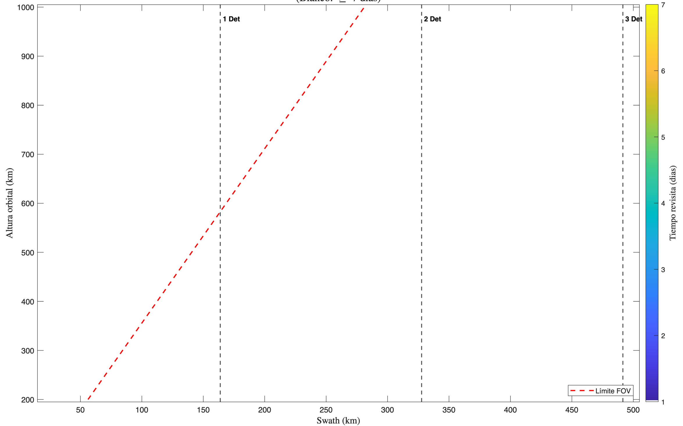
Tiempo Revisita - 1 Satelite(s); 2 Telescopio(s): TMA; Detector 2 (Blanco: \geq 7 dias)
